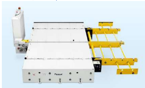
8,000 kN press — 20 ton × 1 die
