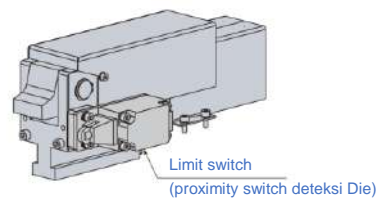
Tipe geser otomatis dengan limit switch (proximity switch deteksi Die)
