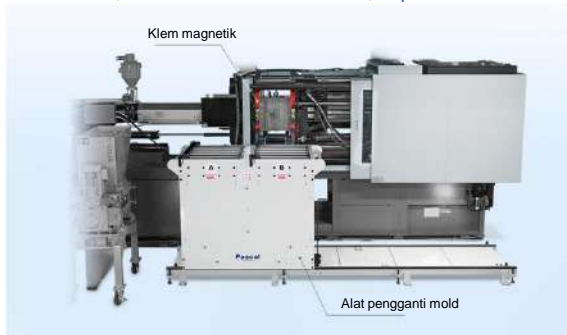
500 kN IMM — Manual, Non track, Tipe Elevasi Meja
