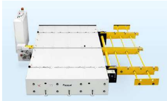
8,000 kN pres — 20 ton × 1 die
